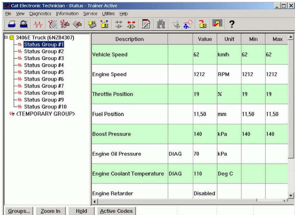
Giao diện phần mềm – Hiển thị thông số kỹ thuật hiện hành
