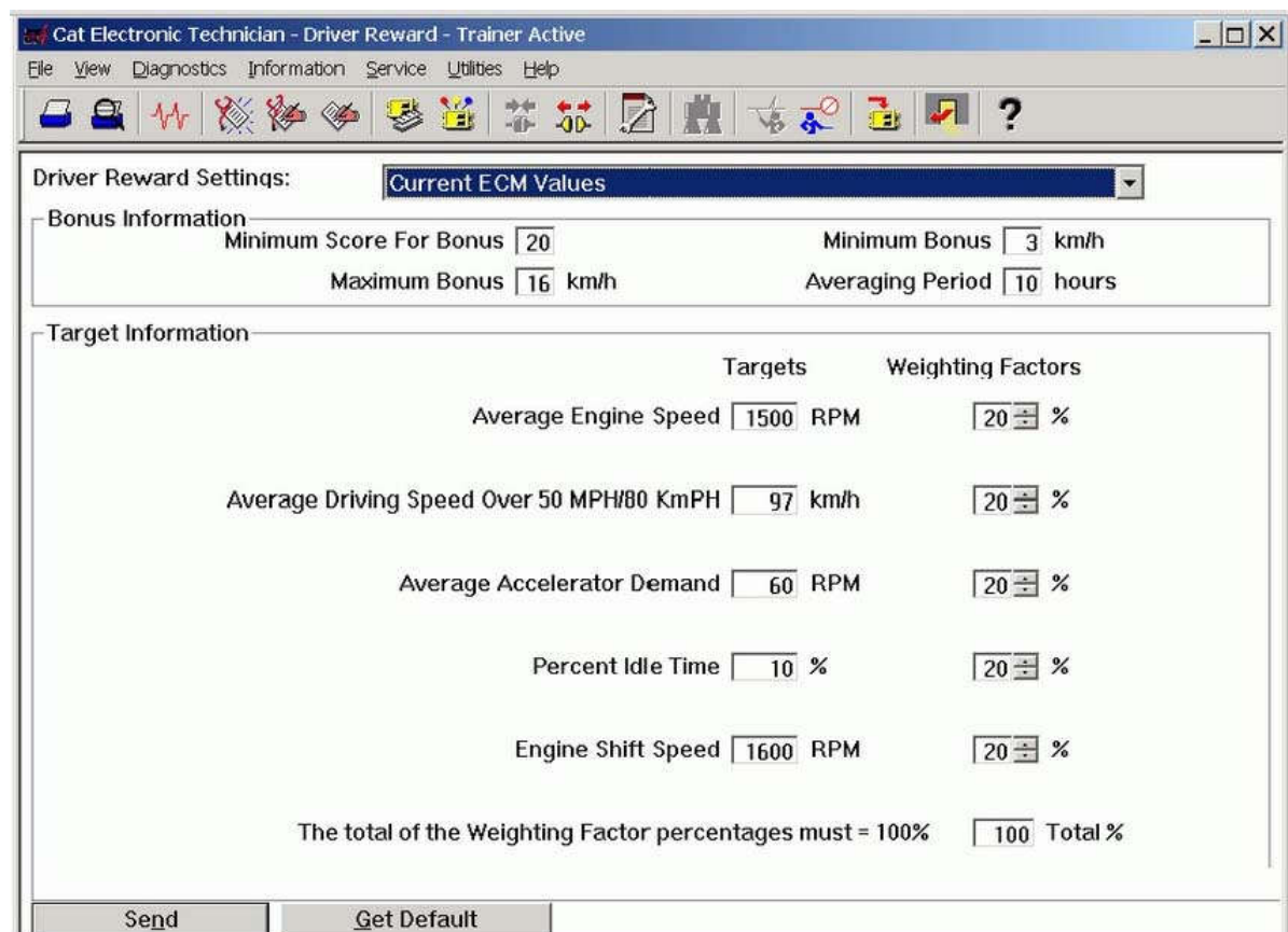
Giao diện phần mềm – Cài đặt, hiệu chỉnh và hiệu chỉnh chuẩn tham số hoạt động của động cơ
